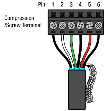
Belden 9773
